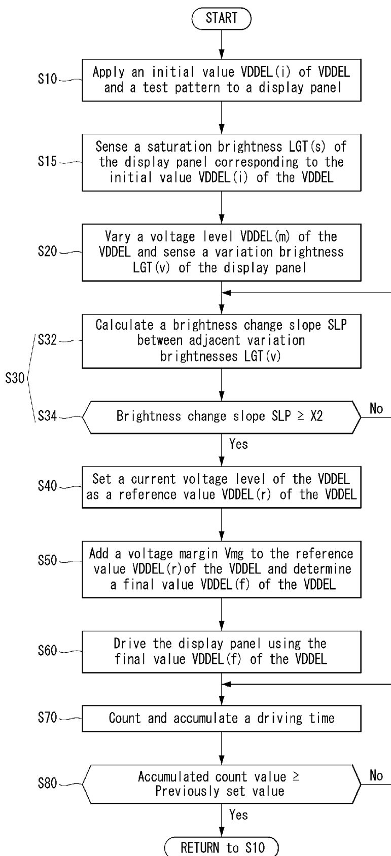
FIG. 16
